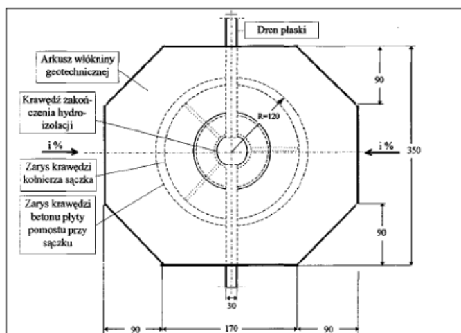
Rys. 5 Szkic szczegółu osadzenia sączka - rzut z góry.
